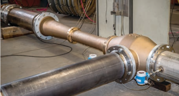
Prüf- und Versuchsstand für die GL-Zertifizierung mit 300er Nennweite
